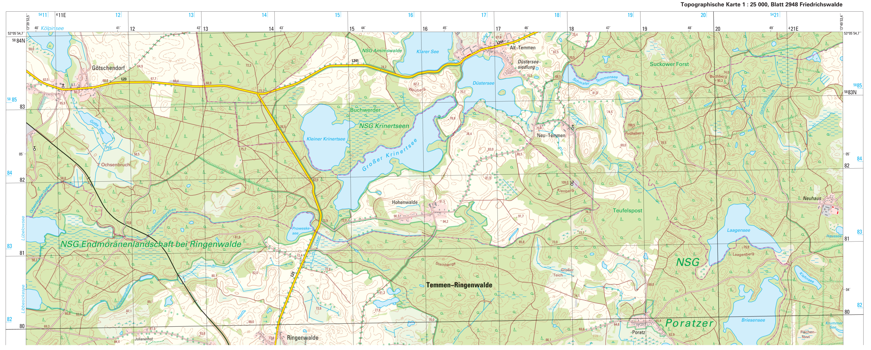
Topographische Karte 1 : 25 000, Blatt 2948 Friedrichswalde
